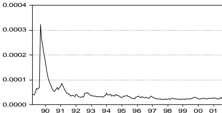
Gráfico 2 Varianza Condicional
